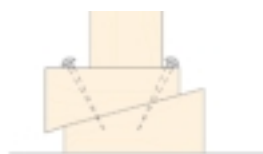
Cunei contrapposti (o biette) per la regolazione in altezza e il disarmo delle centine
