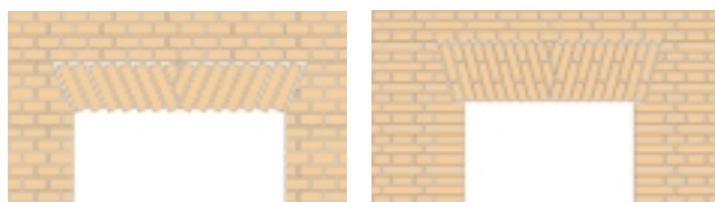
Piattabande alla francese: semplice e a tre teste con semi-incastro alle spalle
