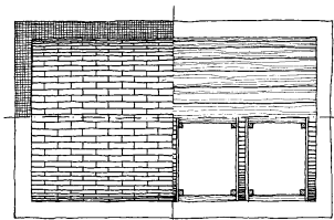
Volte a botte a filari longitudinali
