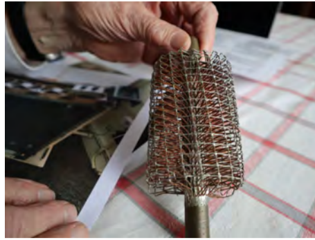
Jón hannaði við annan mann fjölhæfan lághitaofn sem byggir á vatns/lofts-varmaskiptum. Ofninn er með nítján lóðréttum Spirox-varmaskiptum og fimm smáviftum. Hann segir ofninn þann besta sem völ sé á og leitar íslensks framleiðanda.
