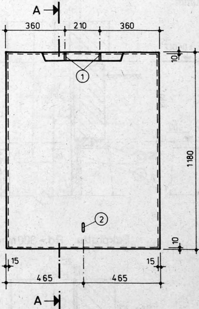
Draufsicht
