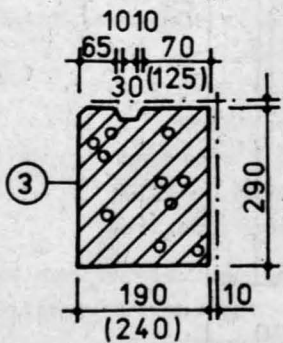
Schnitt D-D
