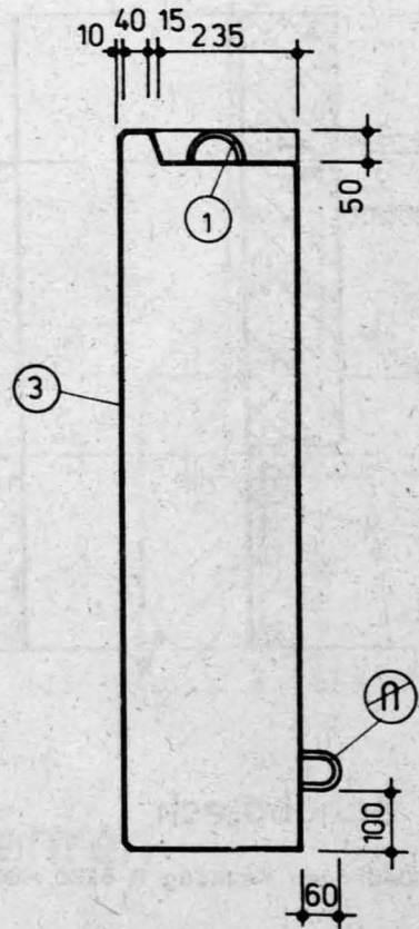
Schnitt A-A
