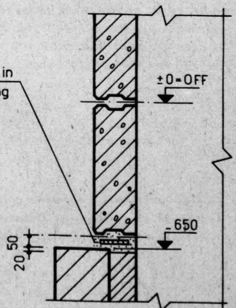
Schnitt B-B
