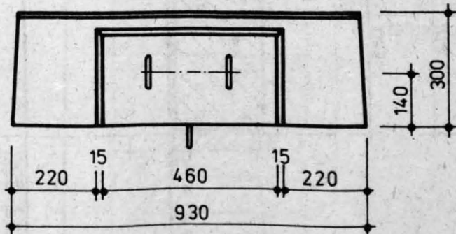
Draufsicht
