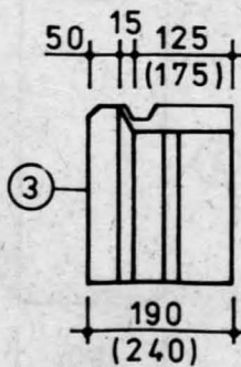
Seitenansicht
