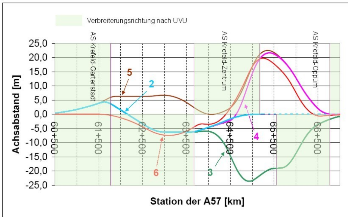
Abb. 2: Gegenüberstellung Achsversätze und empfohlene Ausbaurichtung
