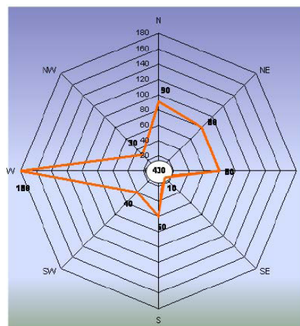
Slika 2.7. Ruža vjetrova
