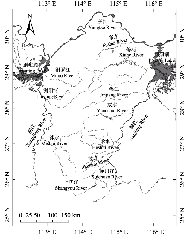
图1 罗霄山脉采样河流的位置示意图
