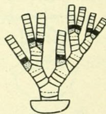
FIG. 15.—ZYGOMETRIDÆ; ZYGOMETRA.
