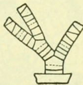
FIG. 16.—ZYGOMETRIDÆ; CATOPTOMETRA.
