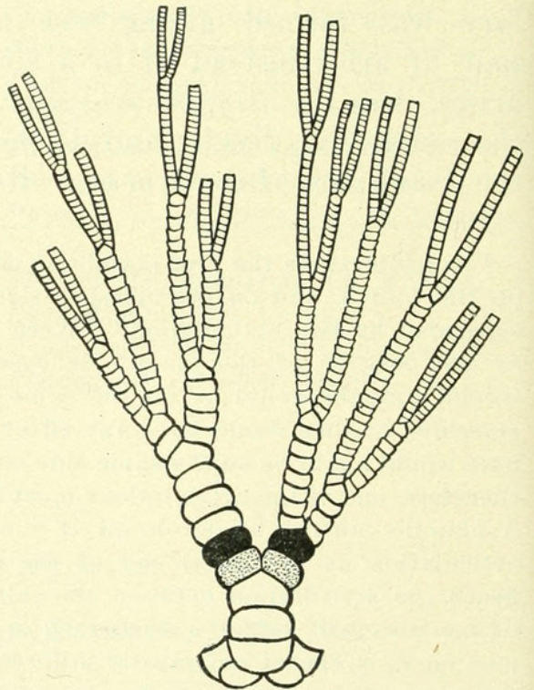
FIG. 27.—PENTACRINITIDÆ; ISOCHRINUS.
