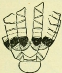
FIG. 17.—ANTEDONIDÆ; HELIOMETRA.
