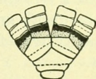
FIG. 22.—COMASTERIDÆ; COMATULA.
