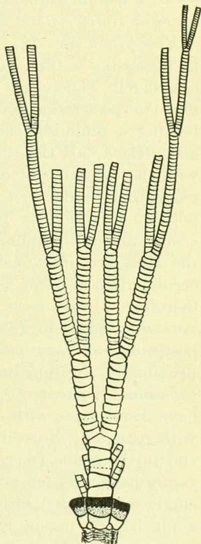
FIG. 28.—PENTACRINITIDÆ; METACRINUS.
