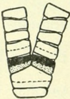
FIG. 21.—COMASTERIDÆ; COMATULA.
