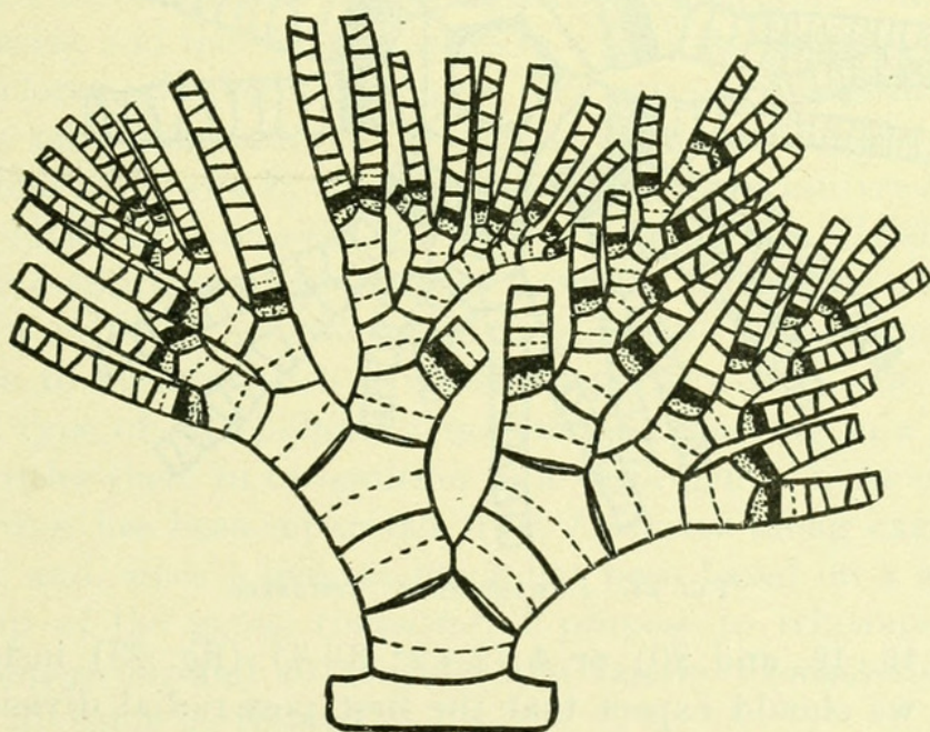
FIG. 23.—COMASTERIDÆ; COMATULA.
