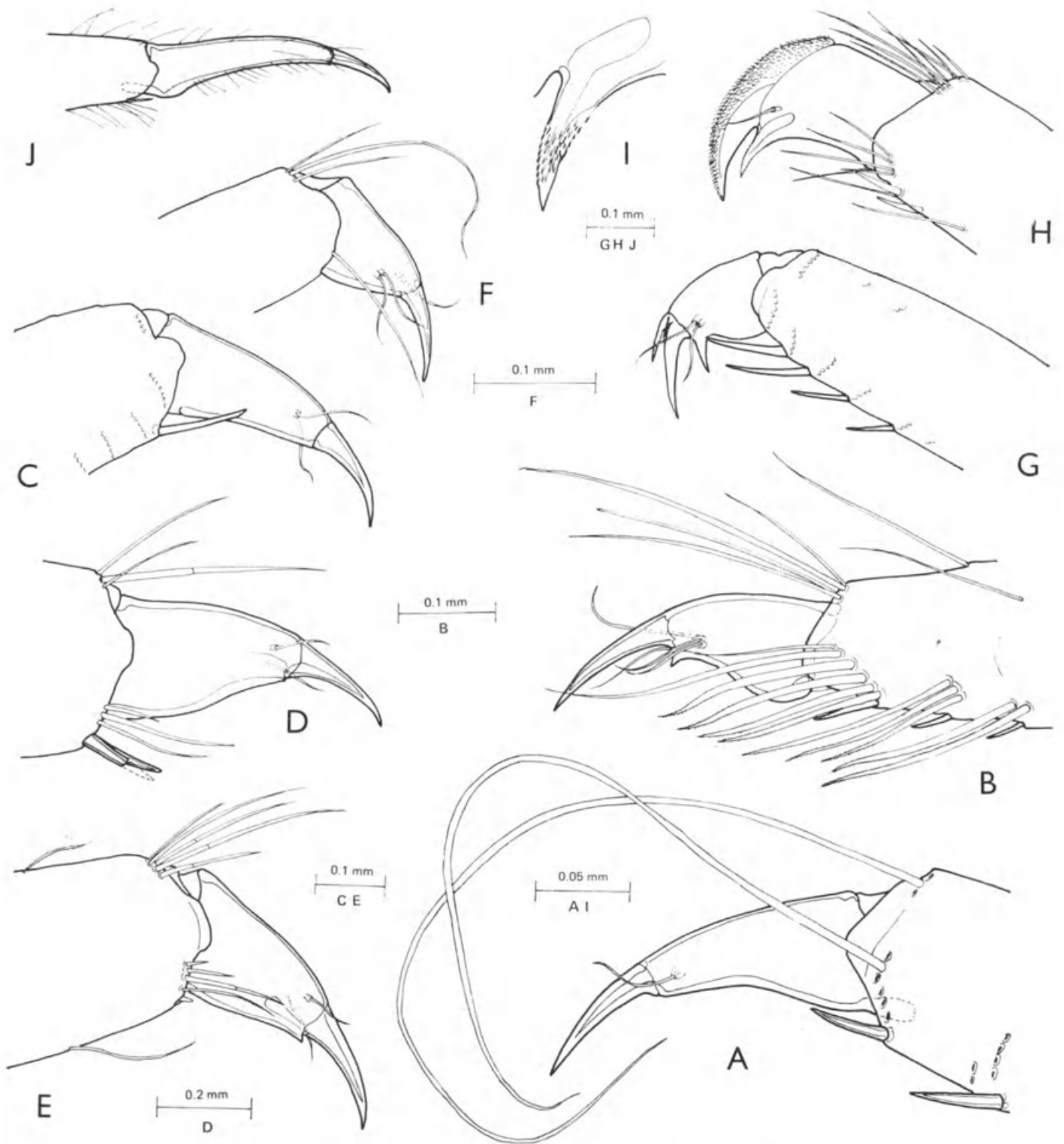
FIG. 7. — Dactyls of third pereiopods : A, Periclimenes affinis (Zehntner) ; B, Periclimenes amboinensis (De Man) ; C, Periclimenes amymone De Man ; D, E, Periclimenes brevicarpalis (Schenkel) ; F, Periclimenes ceratophthalmus Borradaile ; G, Araiopontonia odontorhyncha Fujino & Miyake ; H, Paranchistus serenei sp. nov. ; I, idem , accessory tooth ; J, Pycnodonta hyotis Hipeau-Jacquotte. (A, C, G, propodal setae largely omitted ; B, F, G, ♂ ; D, E, ovigerous ♀.)
