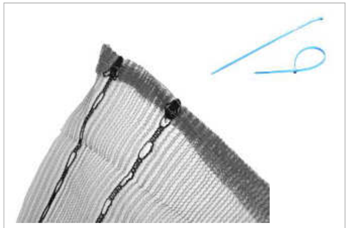
Gerüstschutz-Netz, weiß mit Knopfleiste doppelt verstärkt Nr. 5160187 2,5mx20m Nr. 5160188 3,0mx10m Nr. 5160189 3,0mx20m Nr. 5160175 Gerüstbinder Nylon, 4,8x310 mm, Beutel mit 100 Stk. 16 Nr. 5160177 Gerüstbinder Nylon, 7,8x380 mm, Beutel mit 100 Stk.
