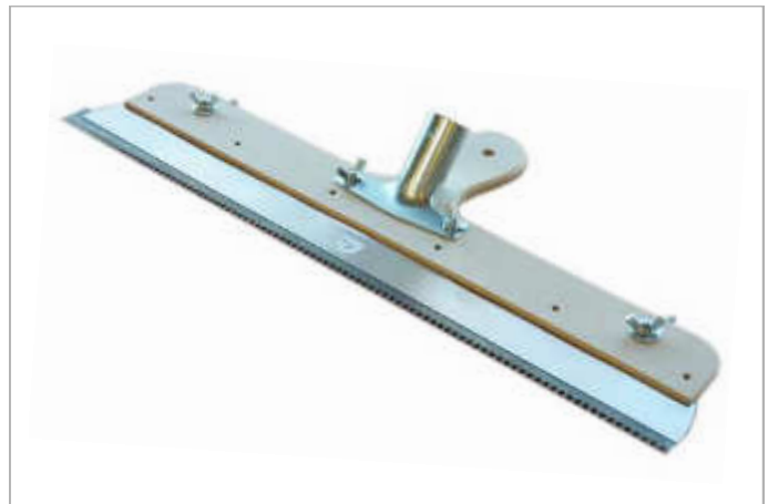
Bodenrakel mit Distanzstiften, rostfrei Für austauschbare Zahnleisten (920131), mit Stielhalter für Holz- oder Teleskopstiel. Mit Distanzstiften zum Einstellen der Höhe Nr. 908632 - 56 cm
