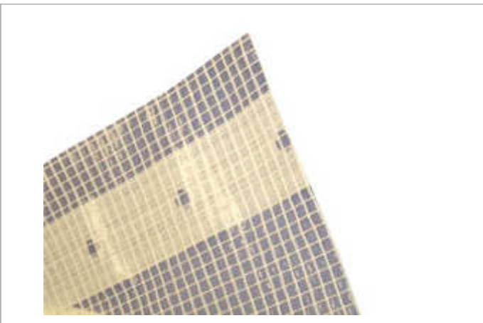
PE-Gittergewebegerüstplane, 170/200gm/m 2 LDPE-Folie mit verstärktem HDPE-Gitter, transparent/weiß UV-stabilisiert, weißes Lochband Nr. 5160180 2,7m x 10m Nr. 5160181 2,7m x 20m Nr. 5160182 3,2m x 10m Nr. 5160183 3,2m x 20m
