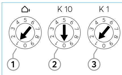
Adressierung Außenstation Trimmer für die Adressierung (Beispiel)
