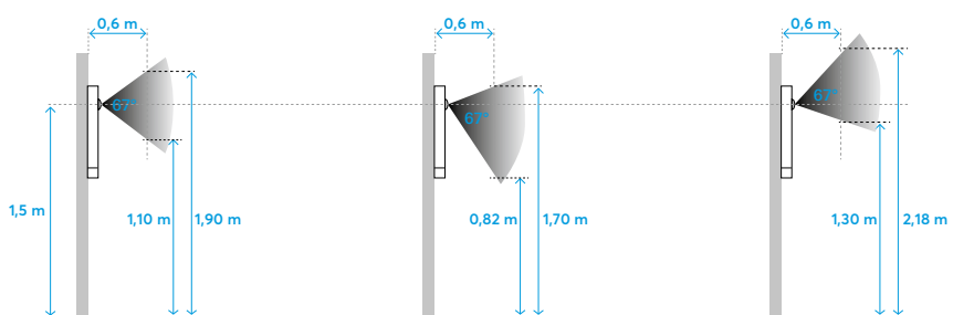
Erfassungswinkel und Einbau-Höhe Kameramodul
