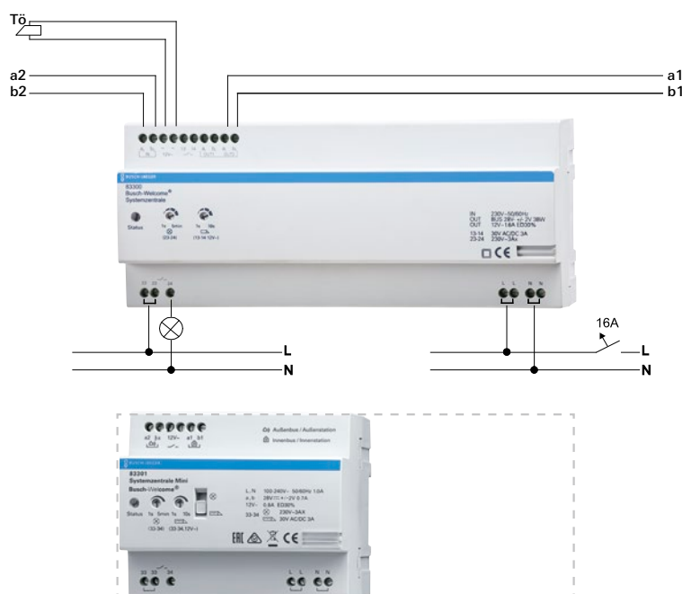
Direkter Türöffneranschluss
