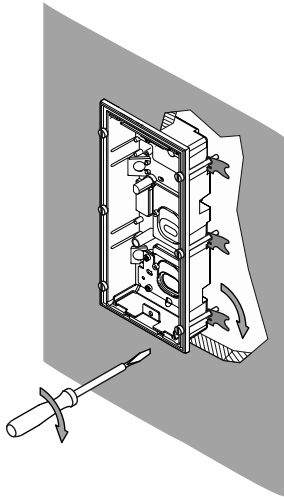
Abb. 86: Montage Montagedosen in Hohlwand: UP-Montagedose klemmen
