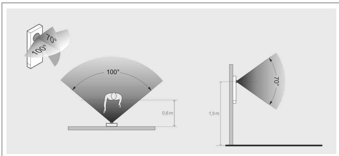
Abb. 26: Erfassungswinkel und Einbauhöhe Audio/Video Modul 130 – A251382M-03
