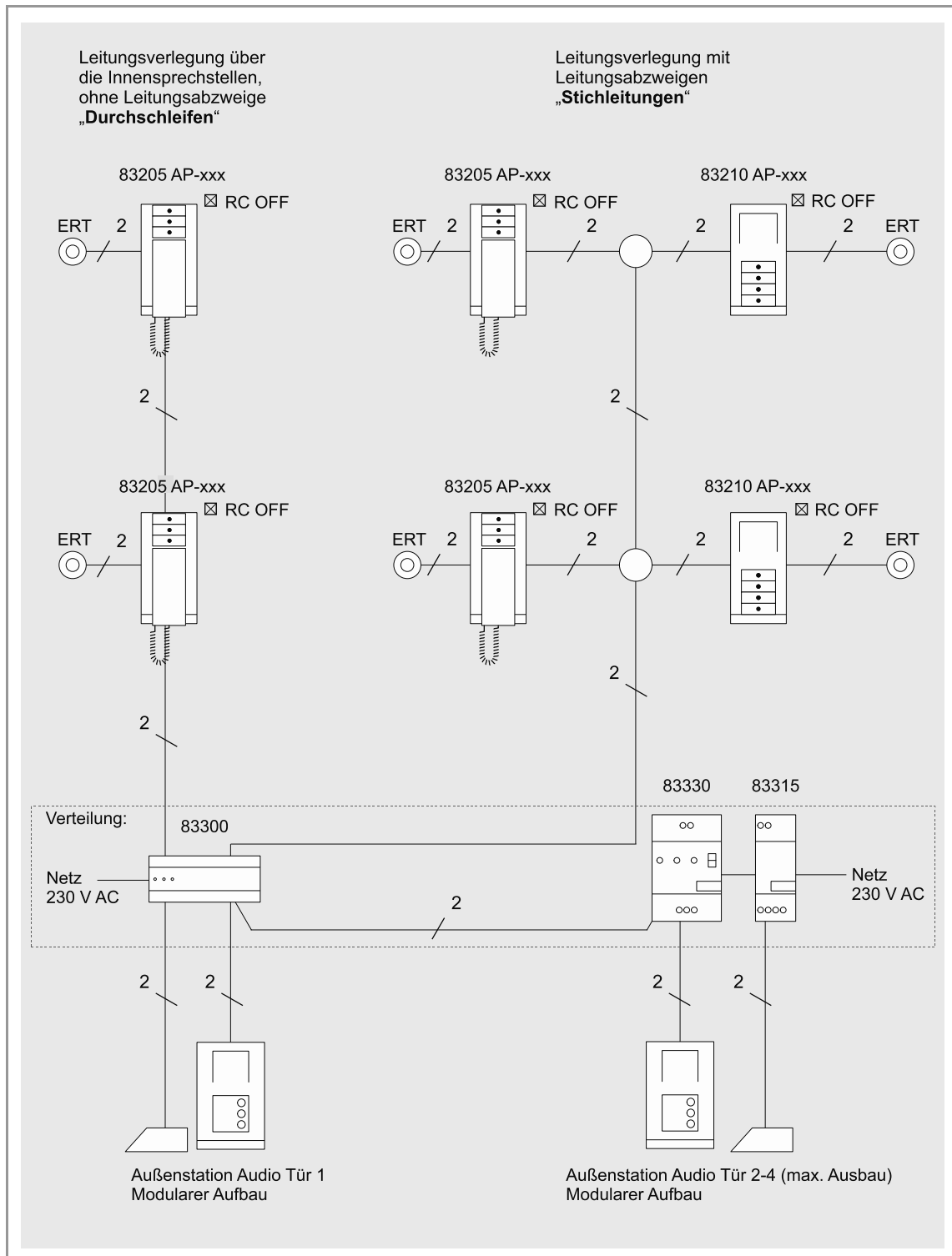
Abb. 19 : Aufbau einer Busch-Wellcome® Audio-Anlage
