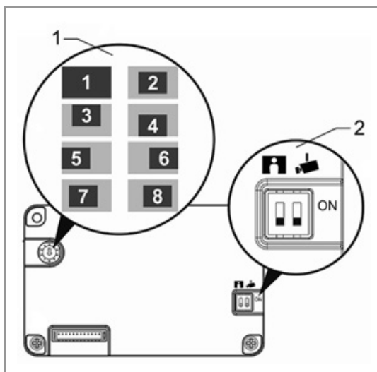
Abb. 24: Einstellung Kameramodul 180°
