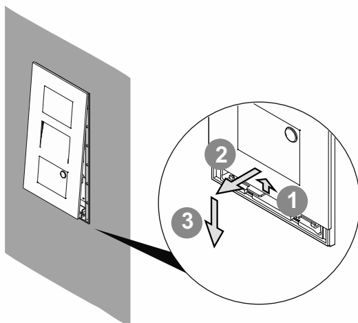
Abb. 90: Montage Außenstation: Gerät abziehen
