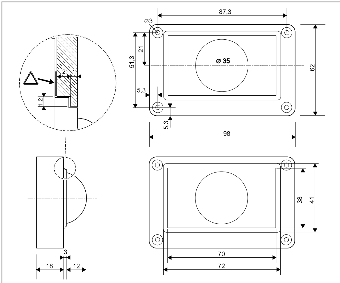
Abb. 97: Maße Kameramodul 83501-101 für bauseitige Briefkastenanlagen
