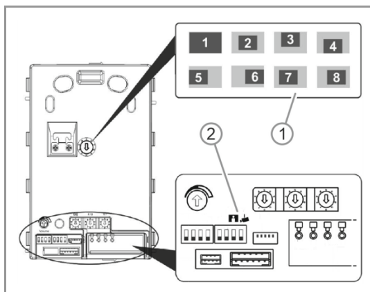
Abb. 28: Einstellung Audio/Video Modul 180
