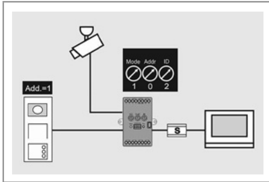
Abb. 64: Kamera Interface Betriebsmodus 1 - Anschlusschema im Außenbus
