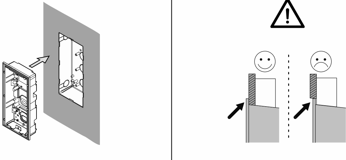
Abb. 82: Montage in gedämmten Fassaden: UP-Montagedose einsetzen
