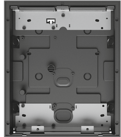
Unterputz-Montagedose Gr. 2/3 41386F-B-03
