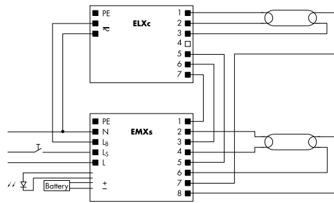
2-lampiger Betrieb – Warmstart mit elektronischem Vorschaltgerät ELXc
