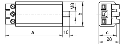
PC-Gehäuse - K D20
