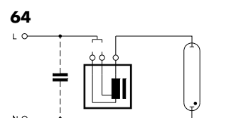
HS-Lampen mit Innenzünder (Vorschaltgerät mit zwei alternativen Spannungsanzapfungen)
