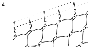
4 X-TEND, Schrägnetz, Montage mit Einzelschlaufen X-TEND, diagonal mesh, Installation with individual loops
