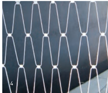
4 Übergroßer Maschenöffnungswinkel, kritische Seilbelastung am Klemmenaustritt, vorrangig für dekorative Anwendungen Oversized mesh opening angle, critical stress on cables at the ferrules' edges, mainly for decorative applications
