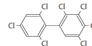
2,2',3',4,4',5,6-επταχλωροδιφαινύλιο
