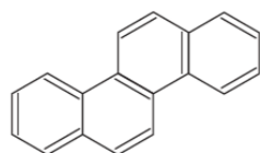
χρυσένιο
