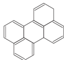
περυλένιο
