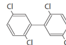
2,2',5,5'-τετραχλωροδιφαινύλιο
