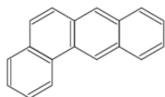
βενζ(α)ανθρακένιο
