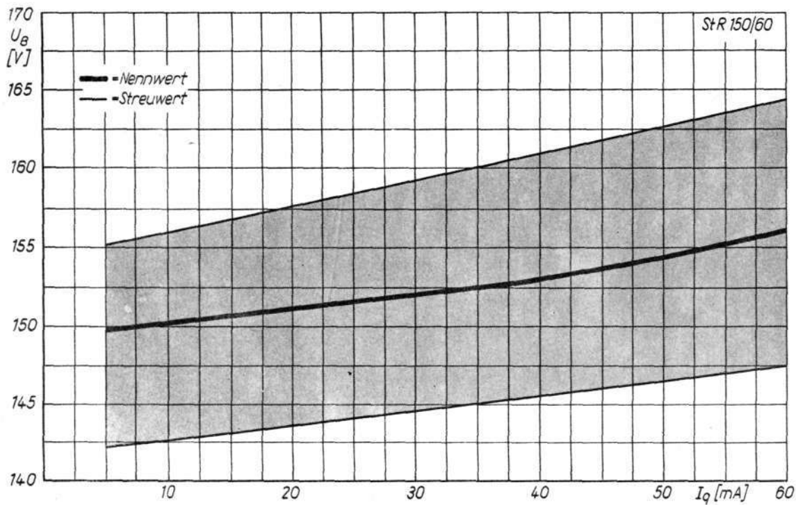
Brennspannungskennlinie
