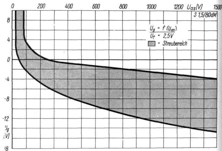
Zündkennlinien-Streubereich
