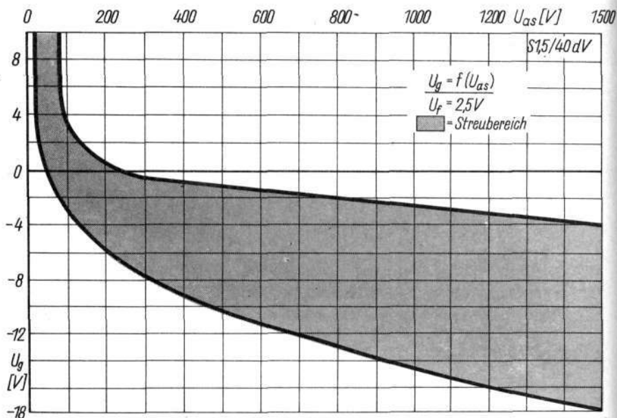
Zündkennlinien-Streubereich
