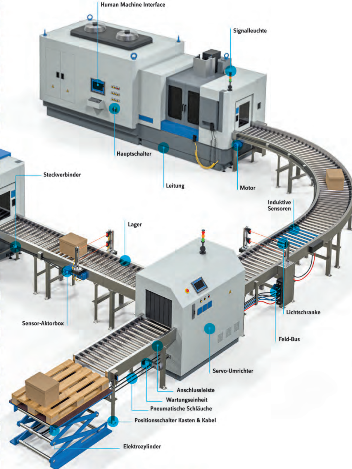
Industriesensoren
