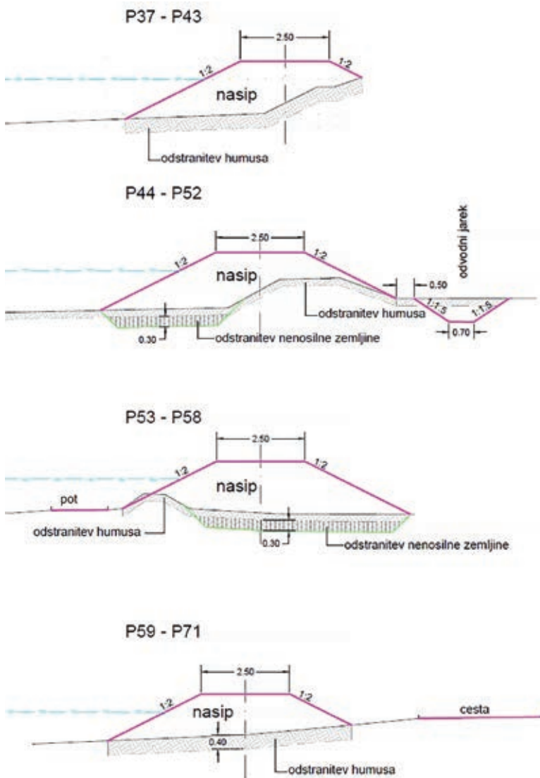
Karakteristični prečni profili (DGD št. 3949/19 VGB Maribor)
