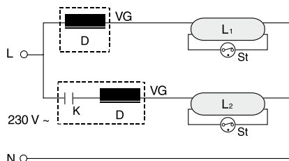
Duo-Schaltung induktiv und kapazitiv (Starter RS 11, 71)
