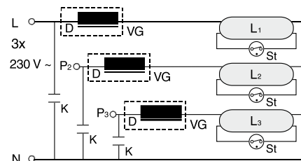
Drehstromschaltung (Starter RS 11, 71)
