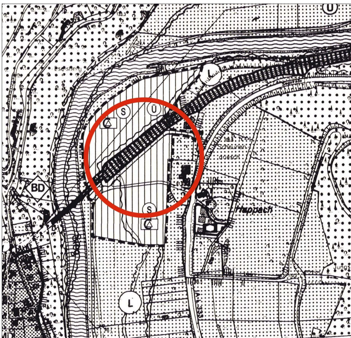
Abbildung 7: Ausschnitt aus dem wirksamen Flächennutzungsplan der Gemeinde Eitorf in der Fassung der 29. Änderung (schraffierte Flächen = Sonderbauflächen, gepunktete Flächen = Fläche für die Landwirtschaft)
