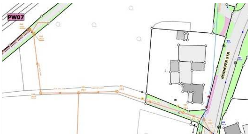
Abbildung 11: Lageplan / vorhandener Kanalanschluss - Quelle: Gemeinde Eitorf
