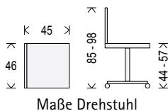
Maße Drehstuhl
