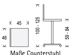
Maße Counterstuhl
