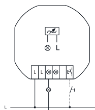
Anschlussbeispiel
