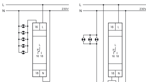
Direkte Ansteuerung der Notleuchten I ≤ 16 A Ansteuerung der Notleuchten über Schaltschütz I > 16 A
