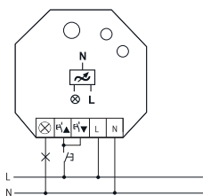
mit Universalstaster
