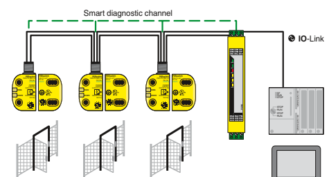
Integrierter Diagnosekanal
