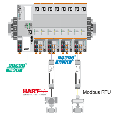
Integration bewährter Feldbusstechnik in PROFINET-Netzwerke
