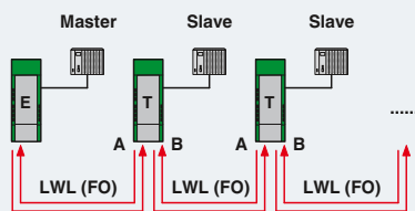
Master-Slave-Linienstruktur
