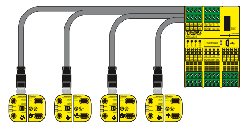
Sichere Einzelverdrahtung
