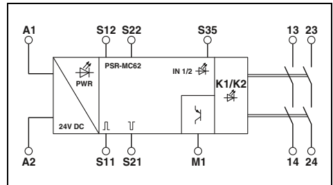
Typ IIIC gemäß EN 574, bis Kat.4/PL e nach EN ISO 13849-1, SILCL 3 nach IEC EN 62061
