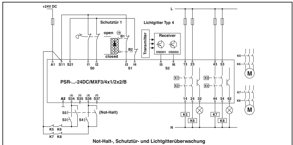
Not-Halt-, Schutztür- und Lichtgitterüberwachung
