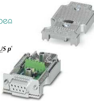
axialer D-SUB-Stecker (Buchse), zwei Kabelzuführungen
