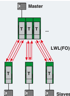
Redundante Sternstruktur
