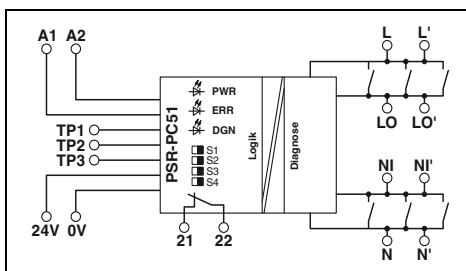
SIL-3-zertifiziertes Koppelrelais zum sicheren Einschalten (F&G), Off- und On-State-Diagnose
