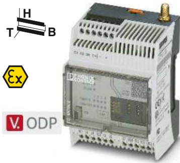
Kommunikation über ODP-Protokoll, 2G-Mobilfunk (GSM/GPRS)
