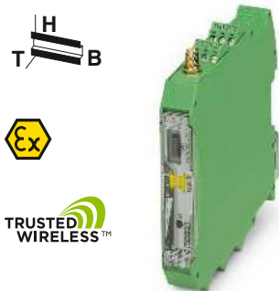
Funktransceiver 868 MHz, für lizenzfreien Einsatz in Europa
