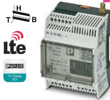
Kommunikation über SMS und E-Mail, 4G-Mobilfunk (LTE)
