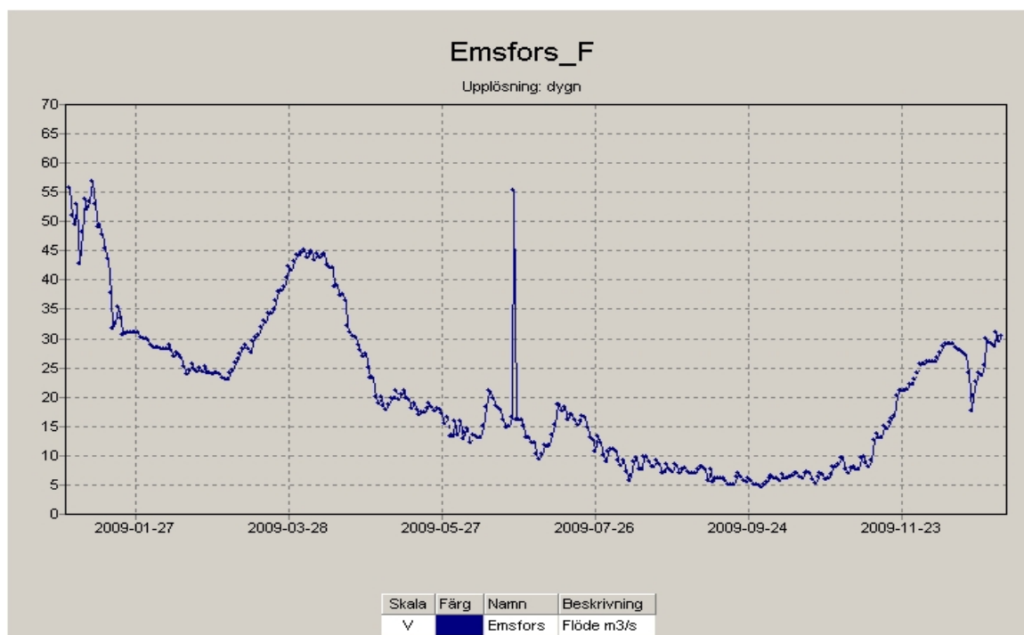
Figur 2. Flödet i Emsfors under år 2009.
