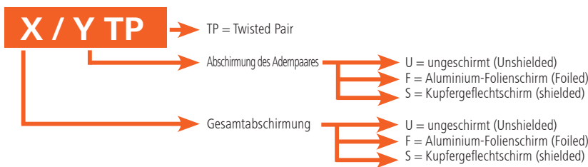
ÜBERSICHTSTABELLE MIT DEN BEZEICHNUNGEN DER NORM ISO/IEC 11801
