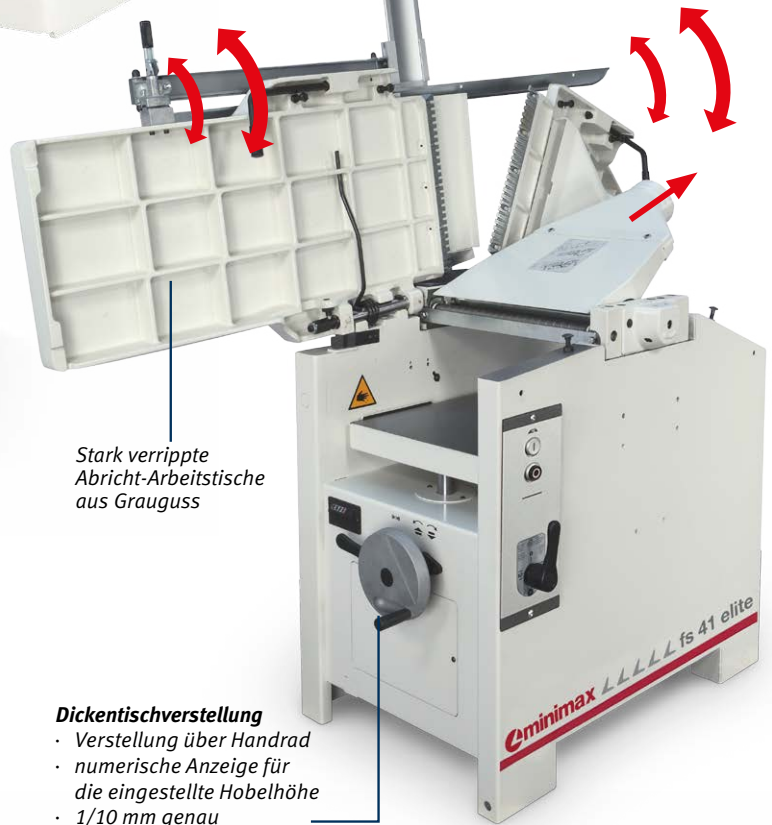
FS 41 elite mit geöffneten Abrichttischen
