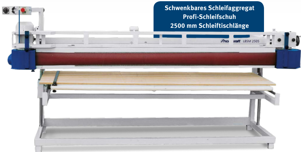
Abb. zeigt LBSM 2505 mit geschwenktem Schleifaggregat als Kantenschleifmaschine
