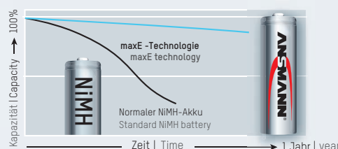
Selbstentladung | Self discharge
