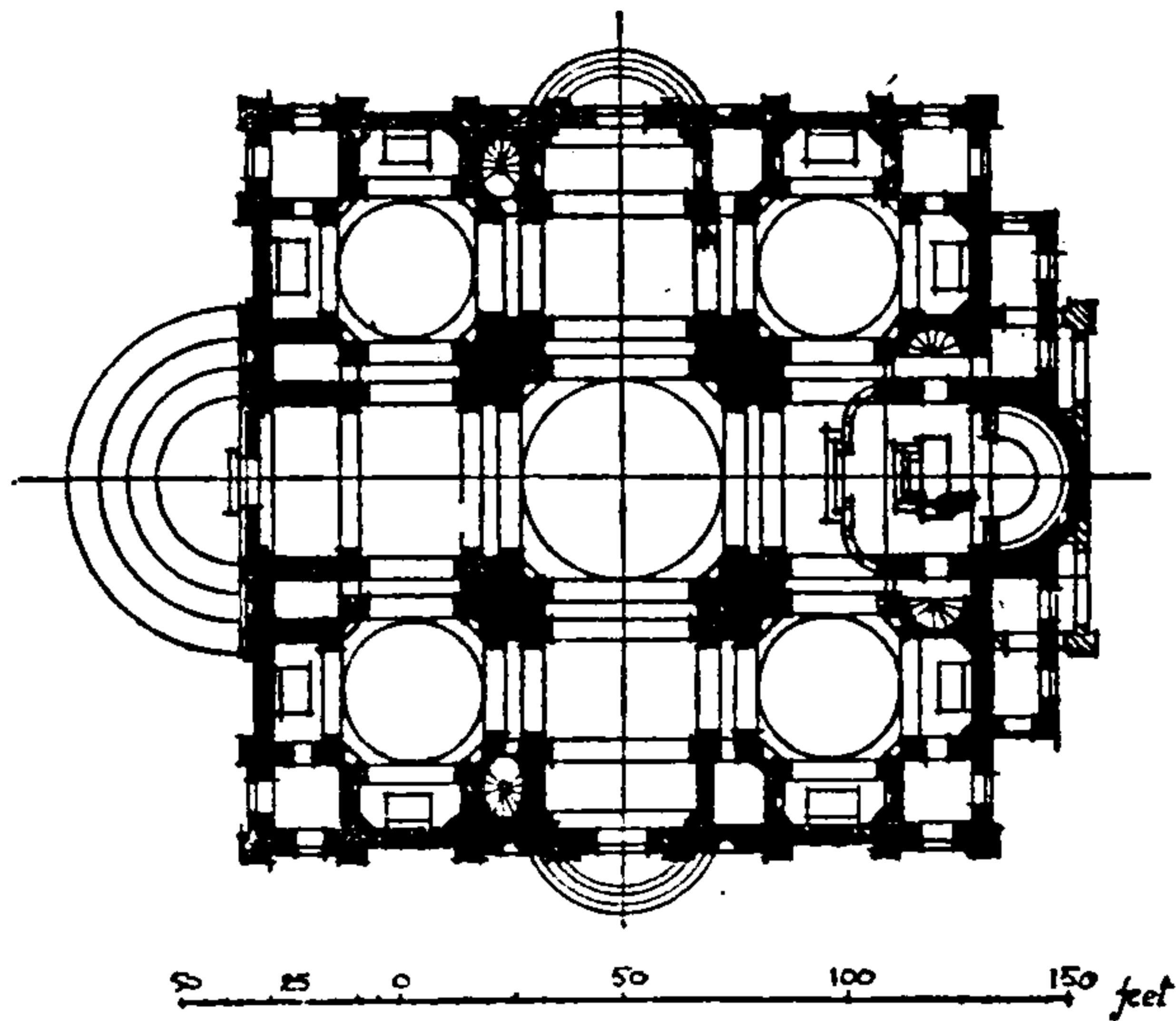
Fig. 21.— S. Maria in Carignano, Genoa. Plan.
