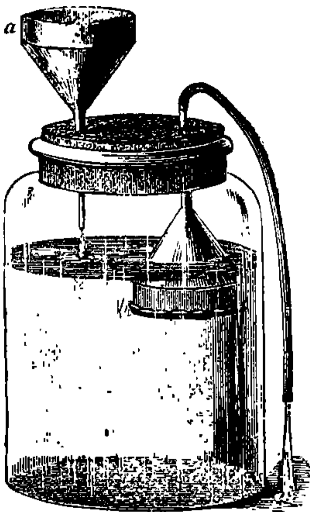
FIG. 3.—FILTERING-BOTTLE
