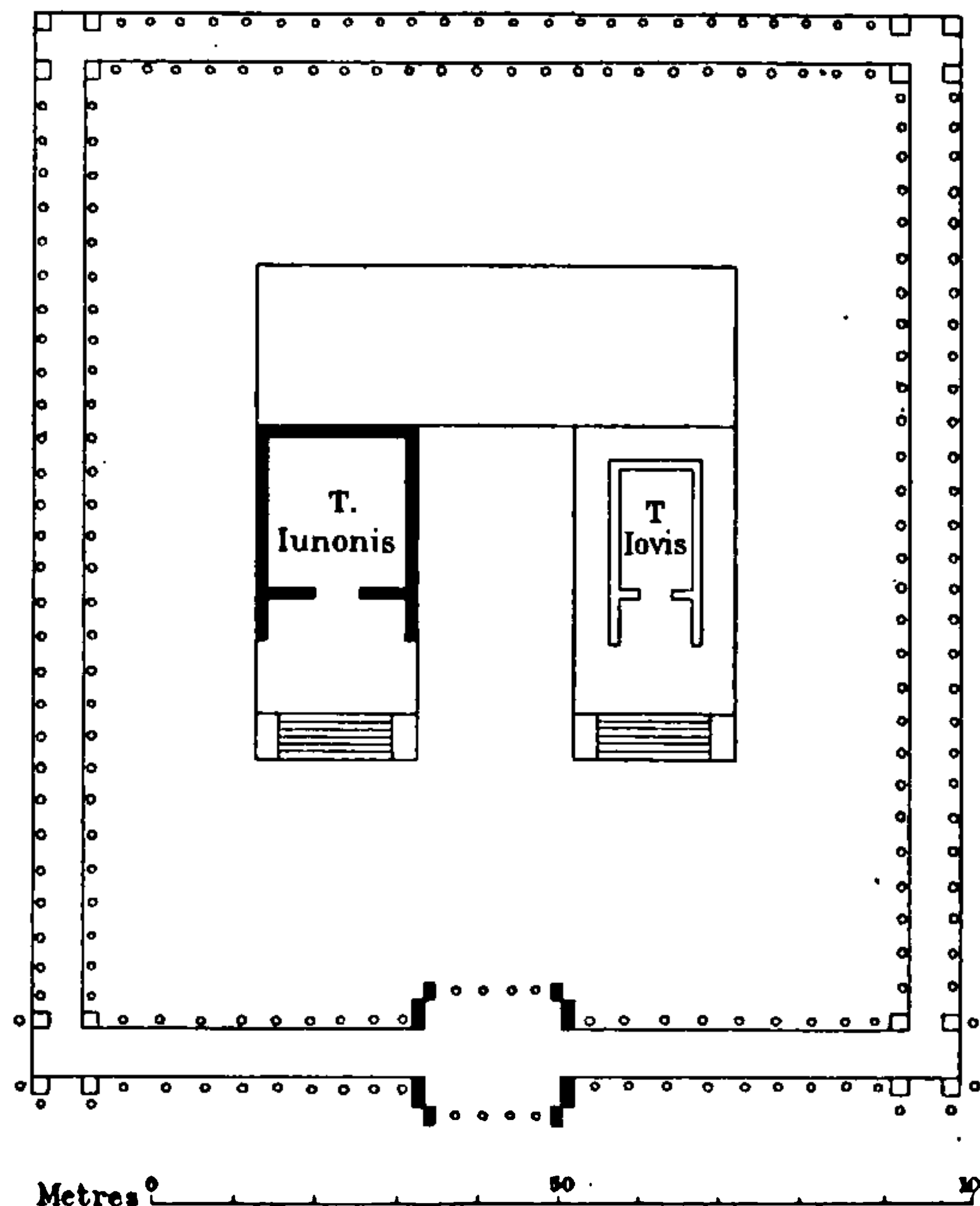
Fig. 3. Plan of the Porticus Octaviae, Rome. From Formae Urbis Romae Antiquae , Berlin, 1896.
