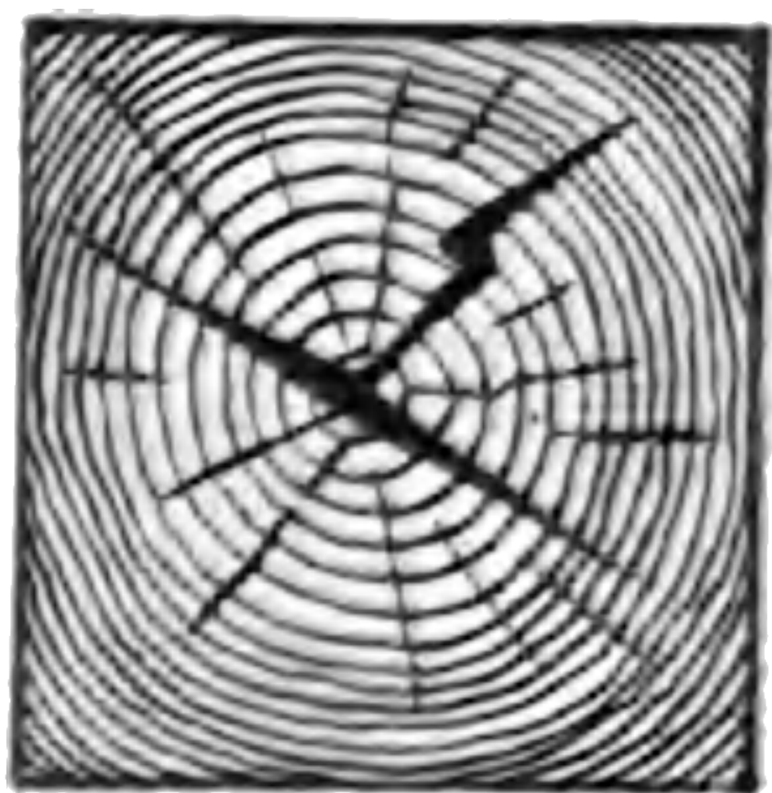
FIG. 42.—Heartshake.
