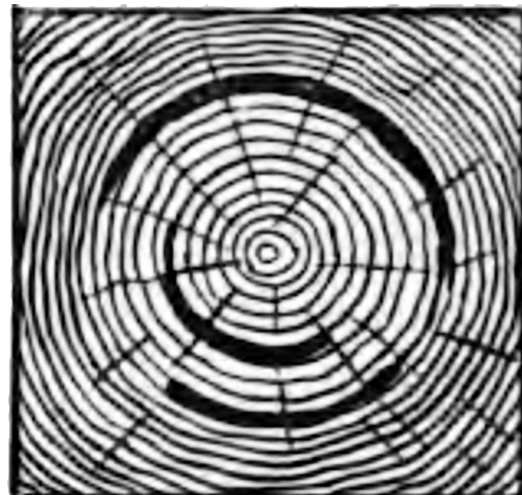
FIG. 46.—Ringshake.
