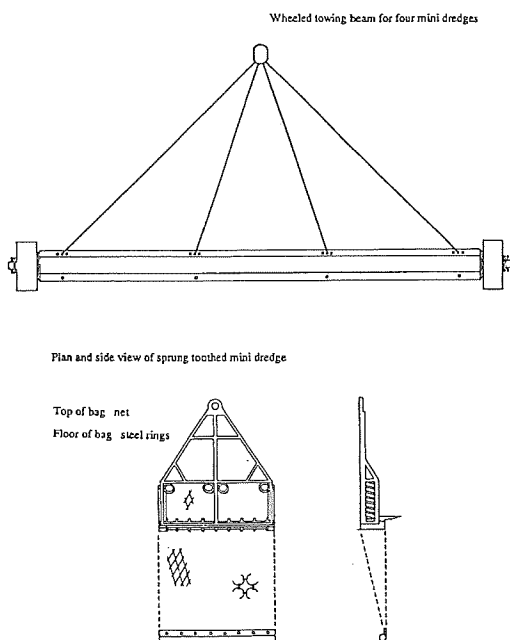
FIG.5. The Scottish mini dredges.
