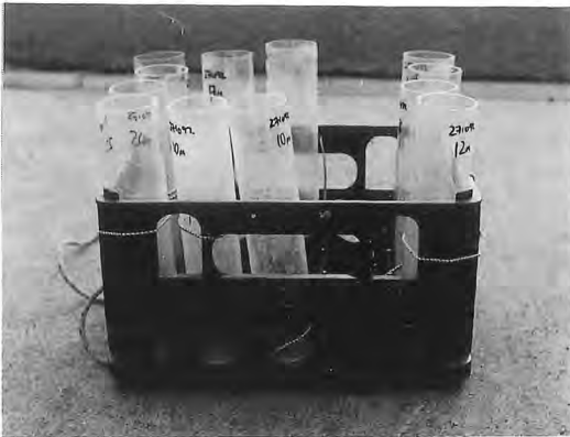
FIG.4. Bed sediment trap.
