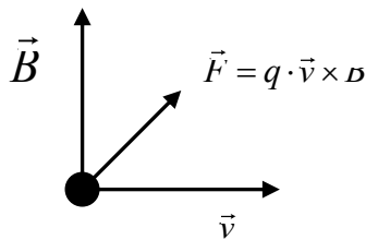
Abbildung 2.3 Kraft auf eine bewegte negative Ladung im magnetischen Feld
