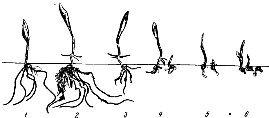
Рис. 1. Влияние гексахлорана на прорастание семян кукурузы:
