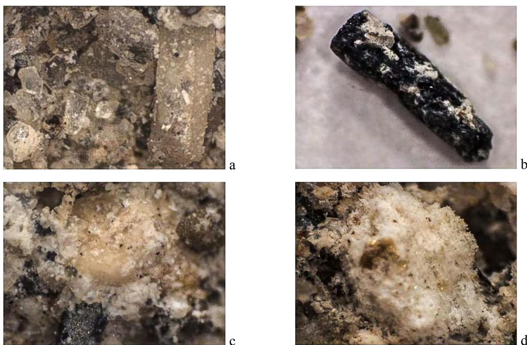
Fig. 3.1.5 - Guado San Nicola: US C. Fasi sialiche (a) e femiche (b) idiomorfe (a, b, c) che si accompagnano a elementi pomice (d) fortemente vacuolari dall'aspetto spugnoso che testimoniano l'assenza di erosione dei componenti vulcanici (foto E. Marrocchino).
