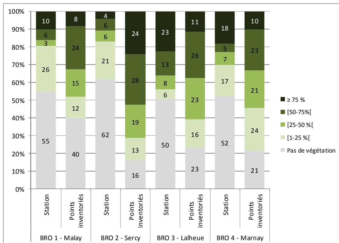
Figure 18: Recouvrement par la végétation des différents points échantillonnés et comparaison avec les points de mesure ayant servi à décrire ces mêmes stations
