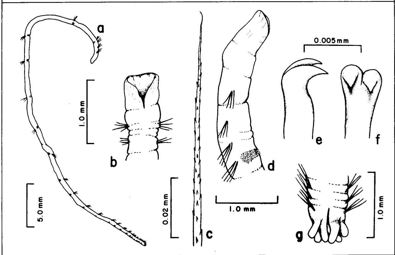
Figure 46-8. Myriochele sp. A: a, whole worm, lateral view; b, anterior end, ventral view; c, notoseta; d, anterior end, lateral view; e, uncinus, lateral view; f, same, frontal view; g, posterior end, dorsal view.
