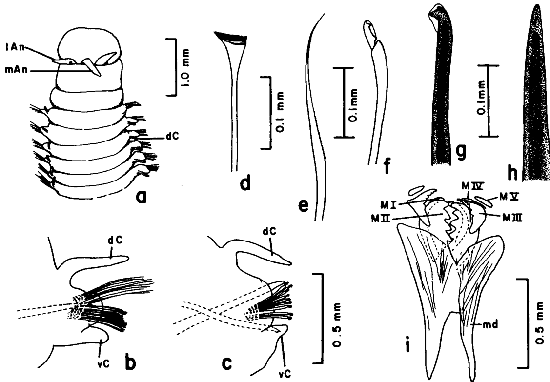
Figure 40-4. Lysidice ninetta : a, anterior end, dorsal view; b, anterior parapodium, posterior view; c, posterior parapodium, posterior view; d, pectinate seta; e, limbate seta; f, compound falciger; g, subacicular hooded hook; h, aciculus; i, mandibles and maxillae, ventral view.
