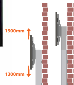
SOPORTE DE PARED REGULABLE EN ALTURA MCSC1301
