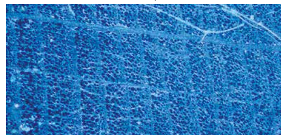
Εγκάρσια τομή σε δείγμα κυπαρισσιού ( Cupressus sempervirens ) από ιστορικό κτήριο στην Κρήτη. Η επιφάνεια έχει λειανθεί και οι δακτύλιοι είναι εμφανείς για παρατήρηση και μέτρηση με χρήση τράπεζας μετρήσεων και στερεοσκοπίου.
