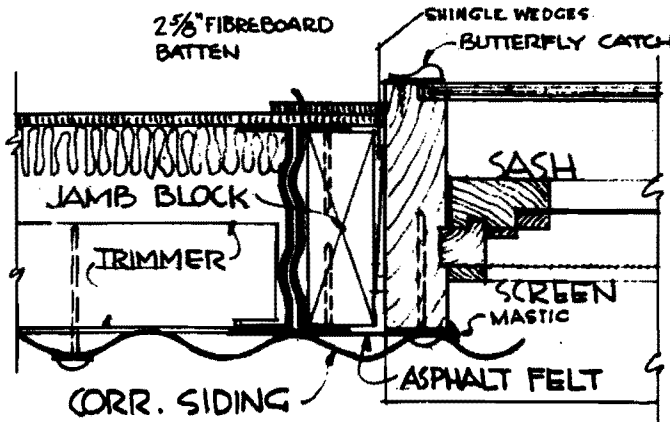
SIDEWALL WINDOW JAMB
