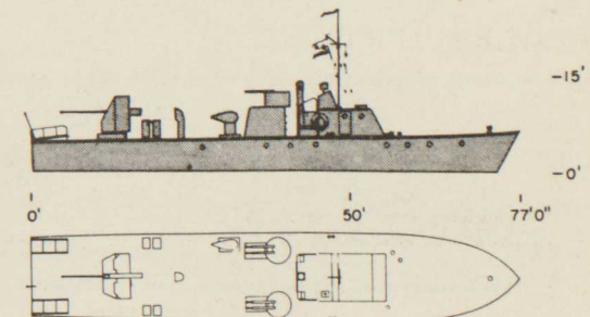
223. "MO VII" CLASS
