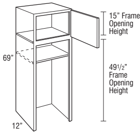
MRSTW18-MRSTW24 L or R
