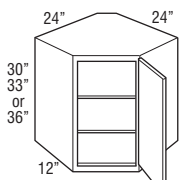
WD2430-WD2436 L or R
