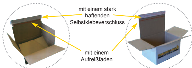
Fefco 703
