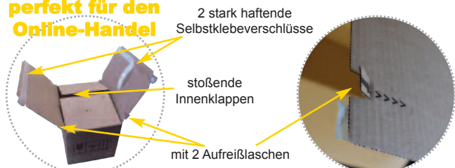
Fefco 703
