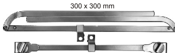
26.3330-10 Rahmen zusammenlegbar Folding frame Cadre pliant Cuadro plegable
