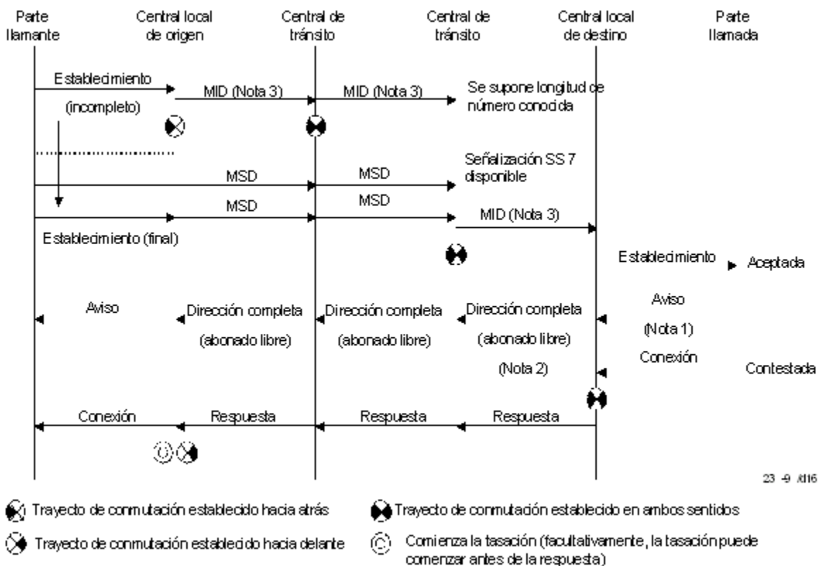
FIGURA D-2/Q.767
