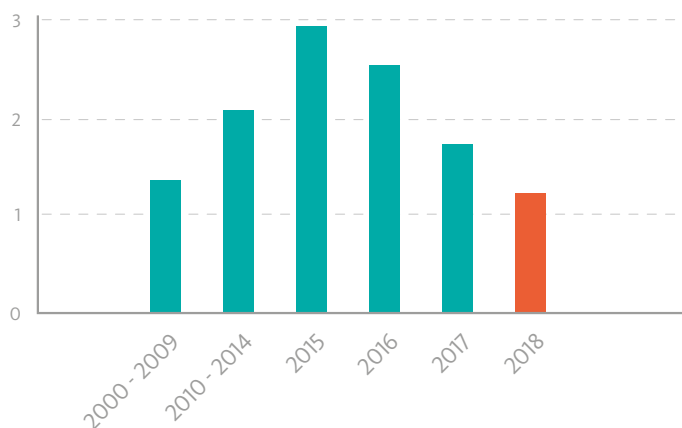
Crecimiento anual (en porcentajes) de la eficiencia en energía primaria, 2000-2018
