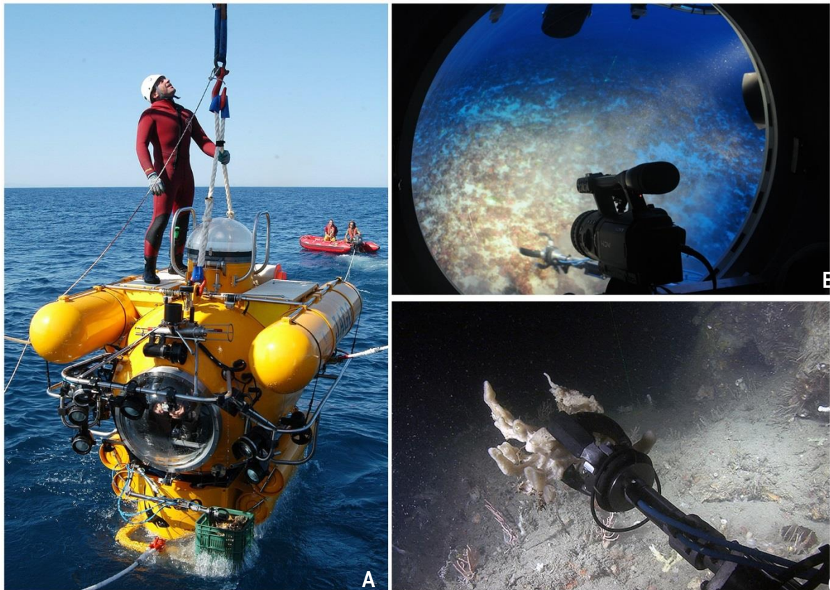
Figura 3.2.3.- El trabajo con un submarino tripulado tiene una serie de condicionantes logísticos particulares y requiere de unas excelentes condiciones de mar. Especialmente críticas son las maniobras de largado y de izado a bordo. Para ambas se requiere la presencia de un buzo profesional (el “hookman”), responsable liberar o asegurar el submarino al cable de la grúa del B.O. una vez que se han comprobado todos los protocolos de comunicaciones y de seguridad (A). El submarino cuenta con una cámara de alta resolución y un brazo articulado (B) que permite la recogida de muestras y su transporte en un cestillo acoplado (C).
