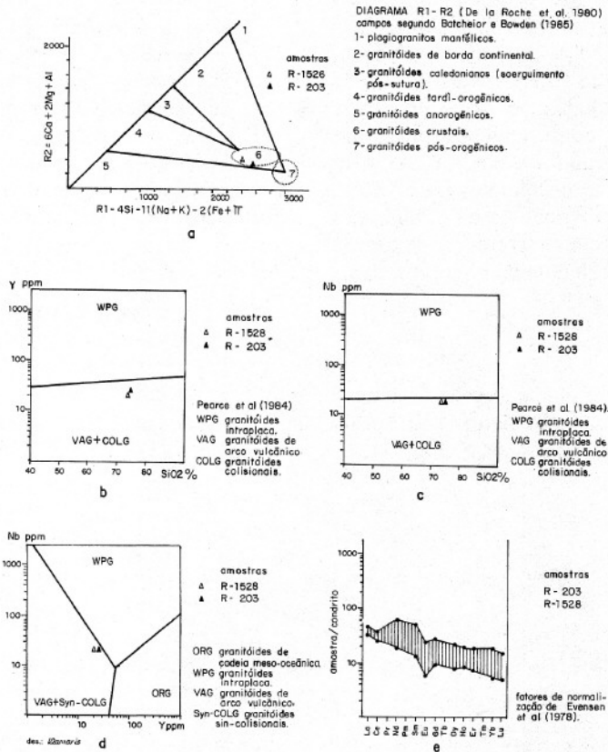
FIGURA 6 - Diagramas petroquímicos.
