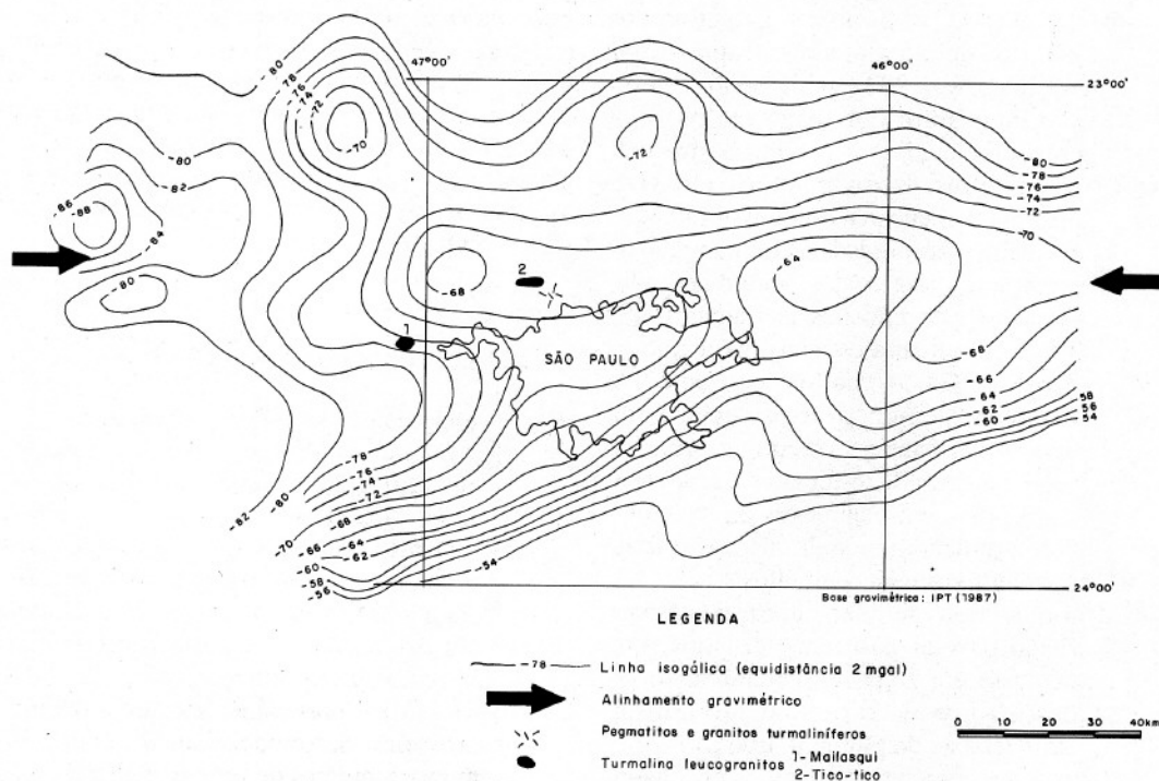
FIGURA 4 - Mapa Gravimétrico Bouguer.
