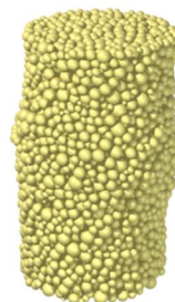
DEM simulations
