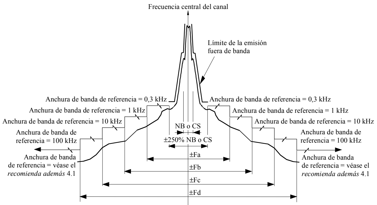
FIGURA 3 Contornos de la emisión no esencial genérica para estaciones del servicio fijo de la Categoría B (véase el Cuadro 11)
