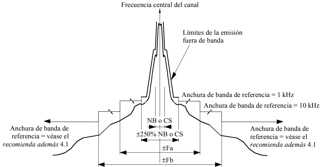
FIGURA 4 Contornos de la emisión no esencial genérica para las estaciones del servicio móvil terrestre de la Categoría B (véase el Cuadro 12)
