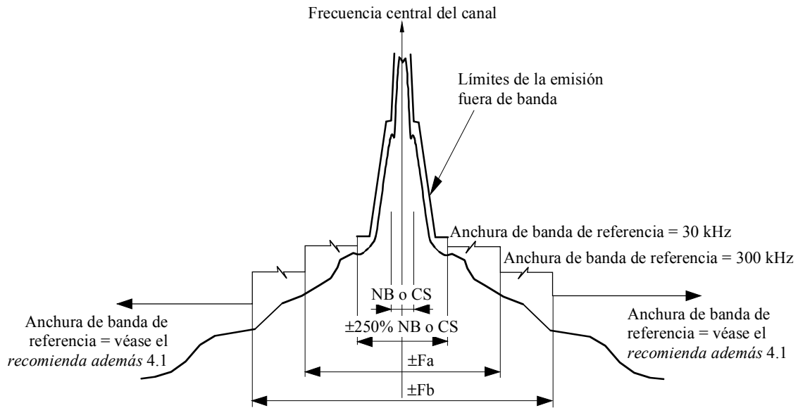
FIGURA 5 Contornos de la emisión no esencial genérica para las estaciones del servicio móvil terrestre de la Categoría B (véase el Cuadro 13)
